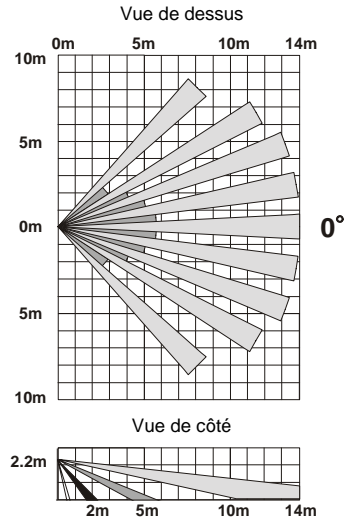
Schéma 2: Zone de couverture lentille standard
